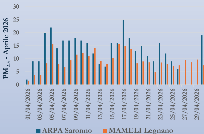
PM 2.5 - Aprile 2026
