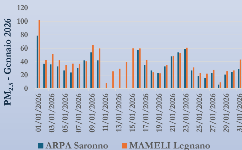
PM 2.5 - Gennaio 2026
